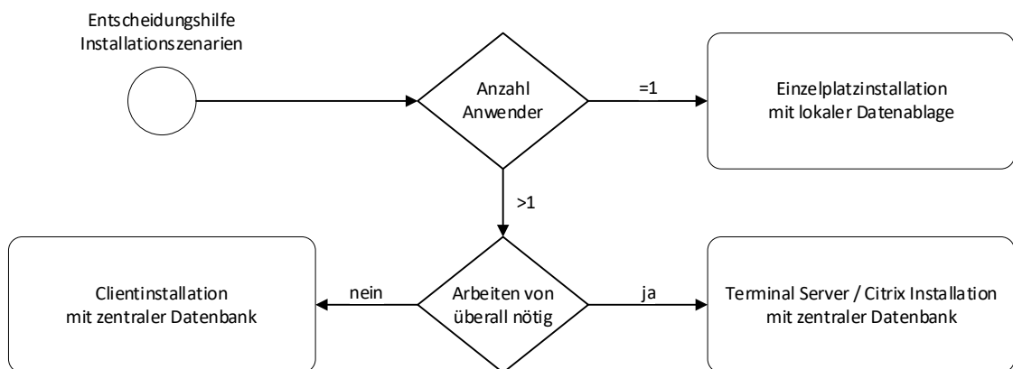
Abbildung 4-1: Entscheidungshilfe Installationsszenario NEVARIS BUILD
