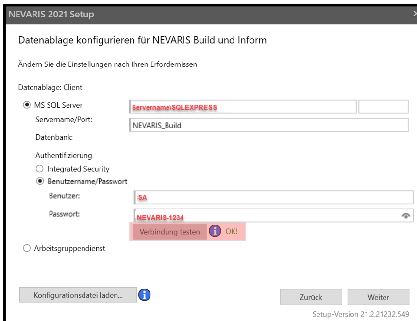
Abbildung 5-24: Setup NEVARIS | Datenablage NEVARIS Build konfigurieren: MS SQL Server Verbindung testen
