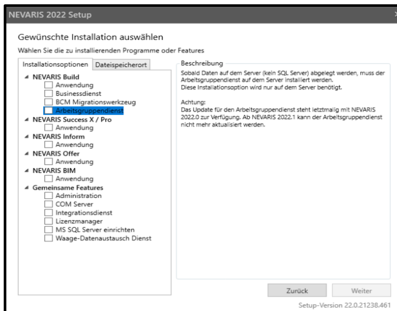
Abbildung 5-4: Setup NEVARIS | Gewünschte Installation | NEVARIS Build | Arbeitsgruppendienst abwählen
