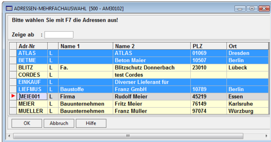
Abb. 8: Mehrfachauswahlfenster
