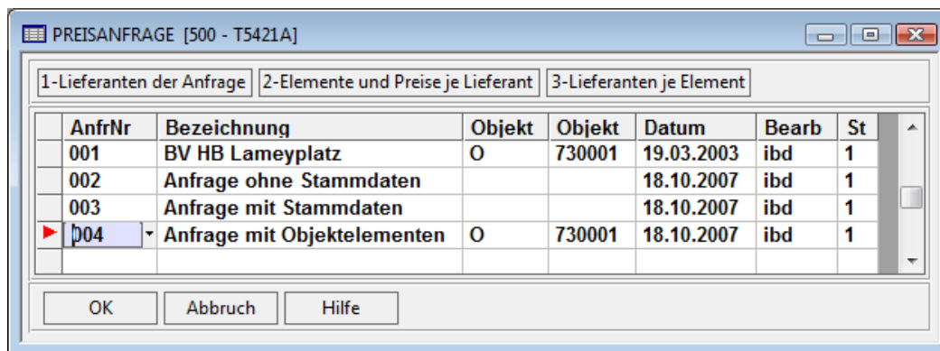
Abb. 9: Hauptmaske Preis-anfrage
