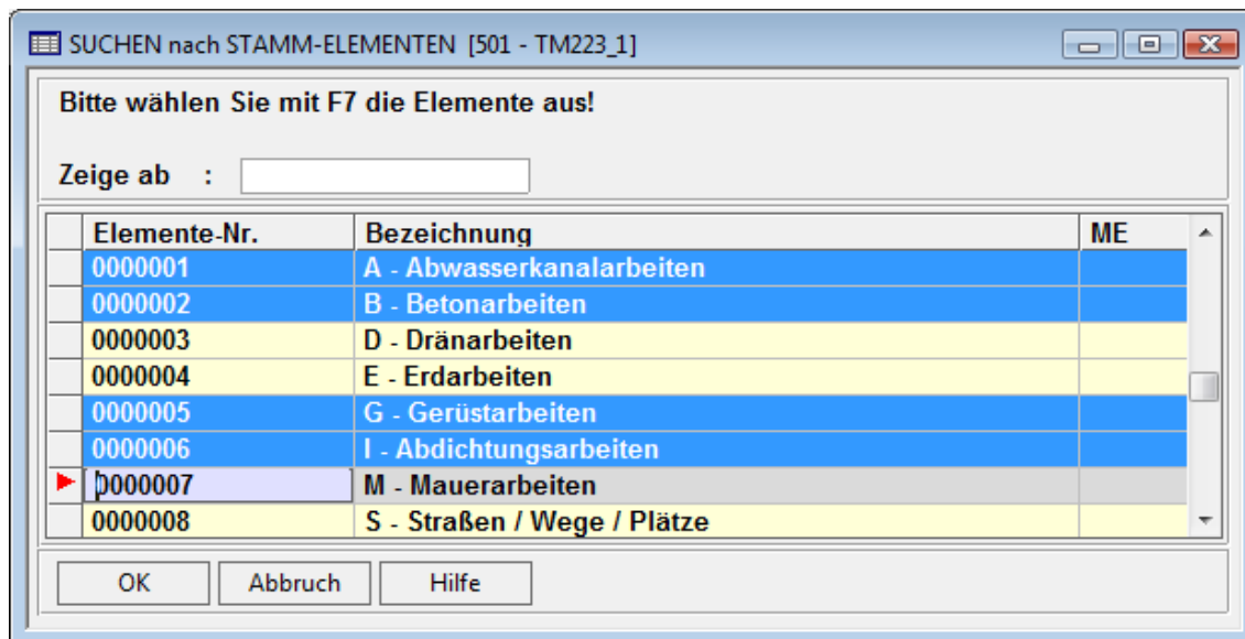
Abb. 22: Auswahlfenster
