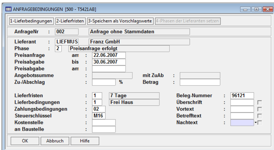
Abb. 4: Anfragebedingungen erfassen
