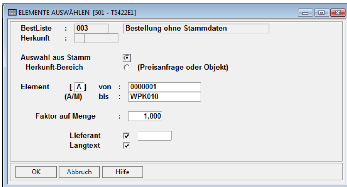
Abb. 21: Elemente auswählen
