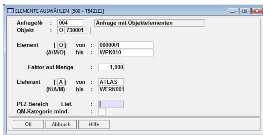
Abb. 10: Objektelemente auswählen
