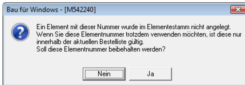
Abb. 20: Hinweismeldung
